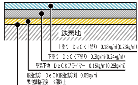
『長期耐候性錆転換防食塗装システム』【NETIS QS-210056-A】
